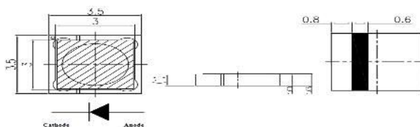
外形图和尺寸
