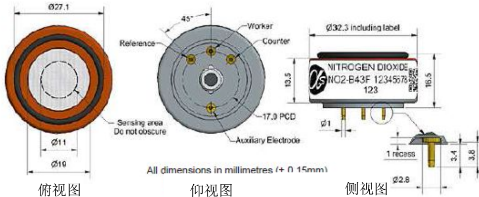
图1 NO2-B43F 示意图
