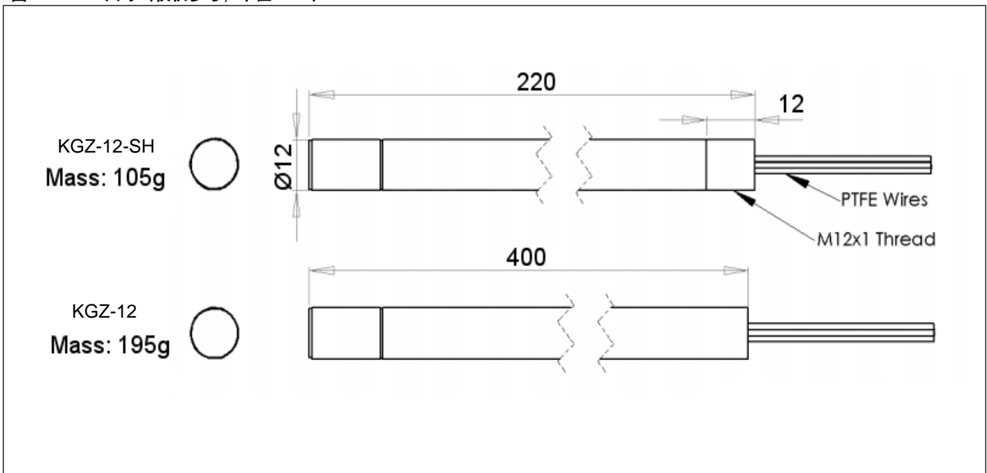
图 1 KGZ-12 尺寸 (仅供参考, 单位: mm)
