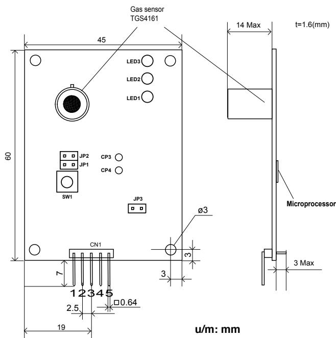
CDM4161 dimensions
