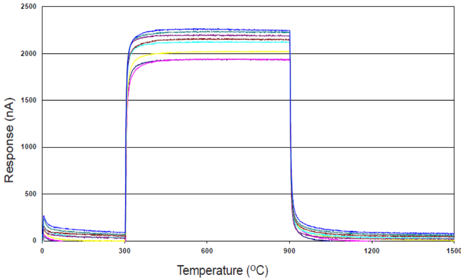
图3灵敏度温度特性
