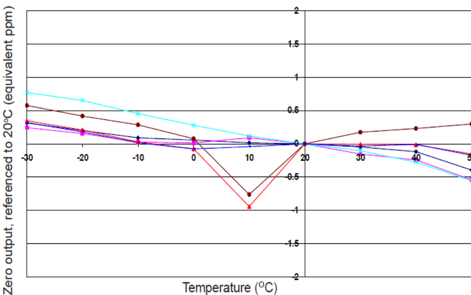
图4 零点温度特性
