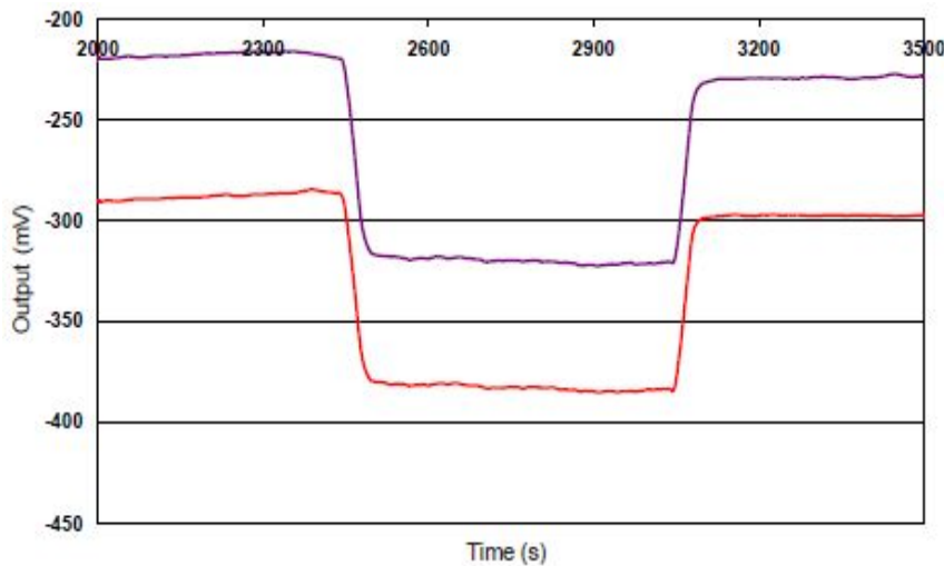
图7 对200ppb NO 2 的反应
