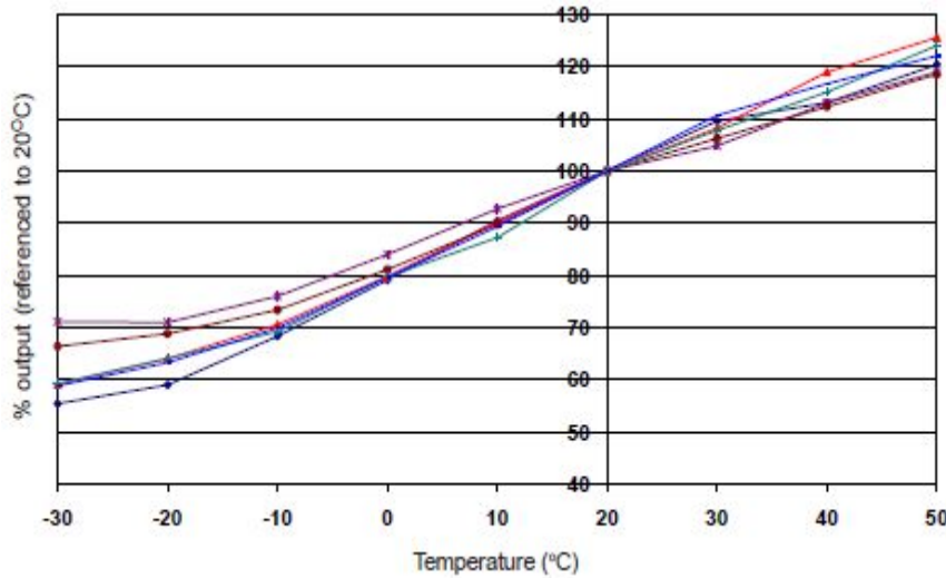
图5 灵敏度温度特性
