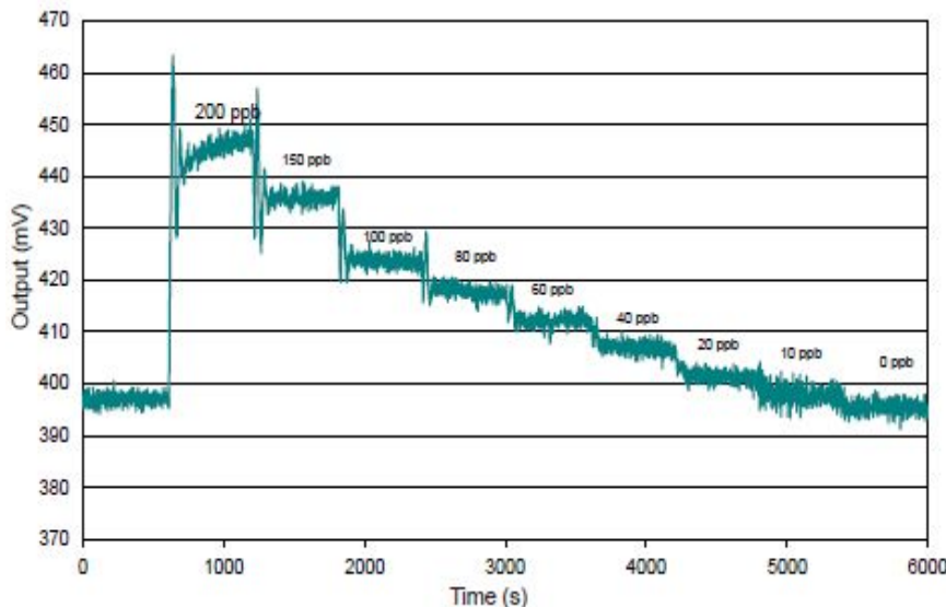
图4 对200ppb O 3 的反应
