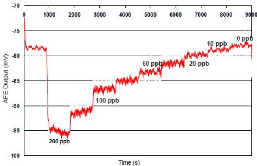
图4 对200ppb NO 2 的反应
