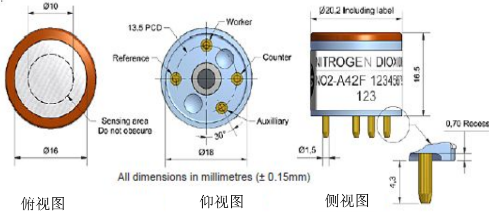
图1 NO2-A42F示意图
