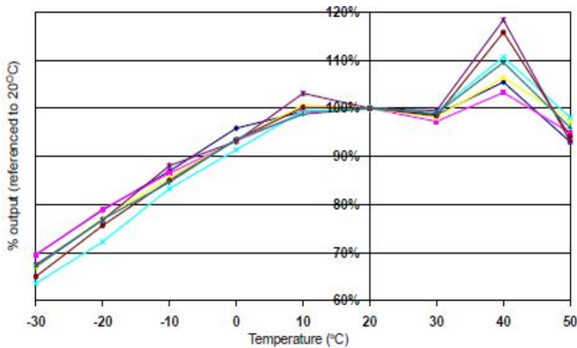
图2 1ppmO 3 时灵敏度温度特性
