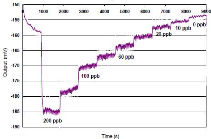
图7 对200ppb NO 2 的反应
