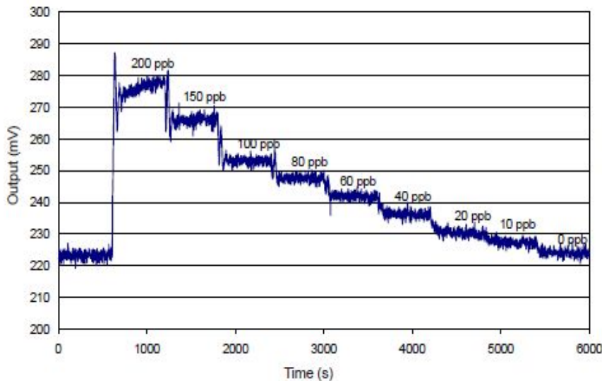
图4 对200ppb O 3 的反应
