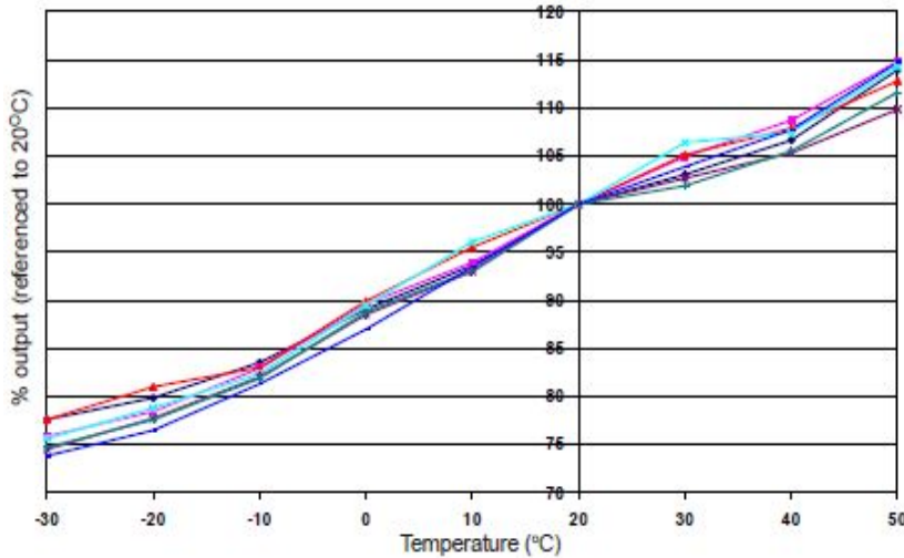
图5 2ppm NO 2 时灵敏度的温度特性
